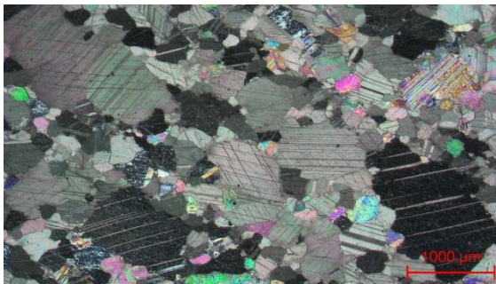
Abbildung 3: Mikroskopische Aufnahme der Marmorprobe aus dem weißen Bereich der Grabplatte im Polarisationsmikroskop, mit dem charakteristischen, ungleichkörnigen ›Mörtel- Gefüge des prokonnesischen Marmors. © Institut für Archäologische Wissenschaften der Ruhr-Universität Bochum, Vilma Ruppene.
